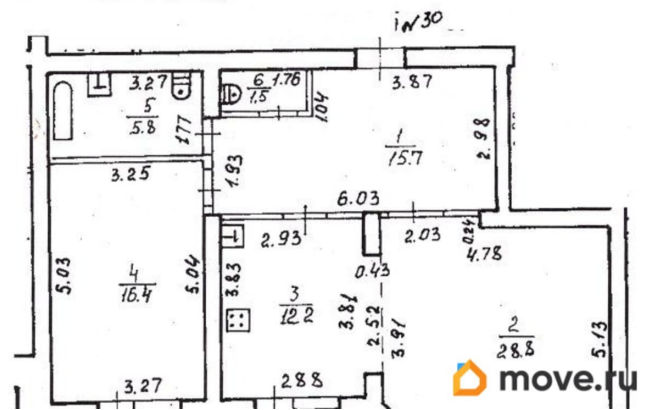
3. План квартиры 30 Масштаб (1 : 100)
