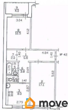
ПОЭТАЖНЫЙ ПЛАН Квартира № 42 (6 этаж) М 1:100
