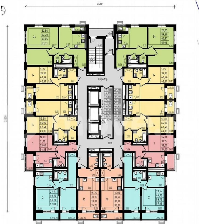
ПЛАН КОМПЛЕКСА "Novaland" . ДОМ ЛИТЕР 10 (квартал 21)
